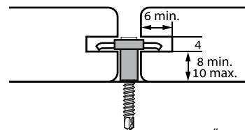
המידות במ"מ
